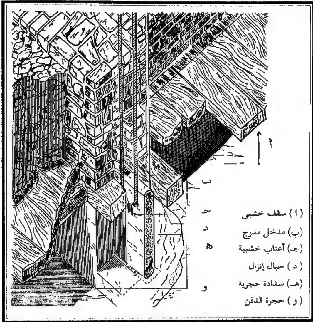
(شكل ٨٤) تفصيل وضع السداة الحجرية في المدخل ذي الدرج
